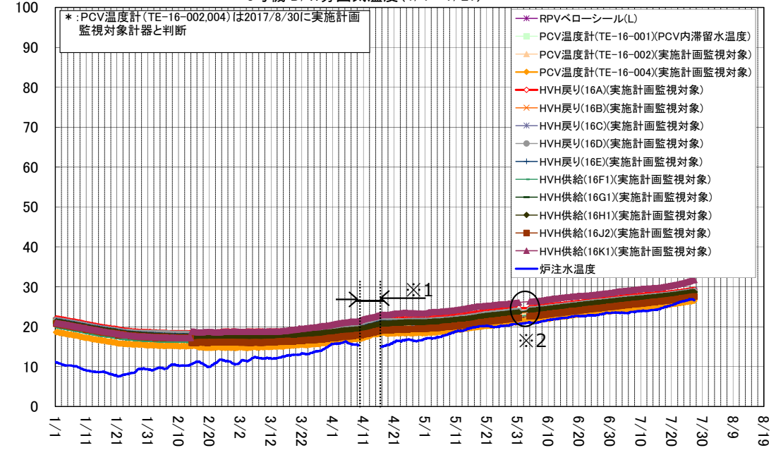
3号機 D/W雰囲気温度(1/1~7/27)
