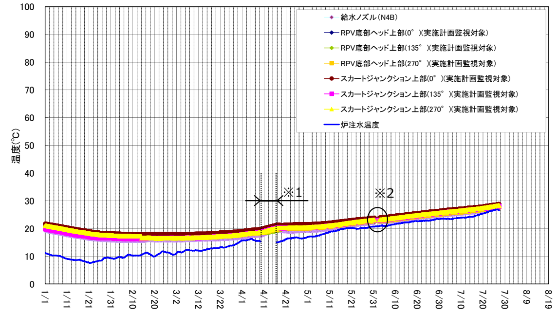
3号機 原子炉压力容器まわり温度(1/1~7/27)
