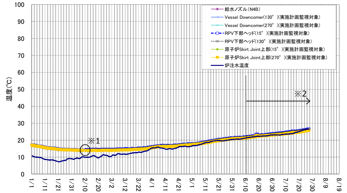
1号機 原子炉压力容器まわり温度(1/1~7/27)
