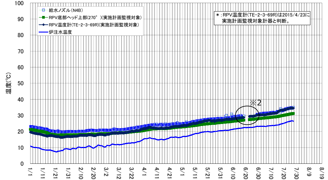
2号機 原子炉压力容器まわり温度(1/1~7/27)
