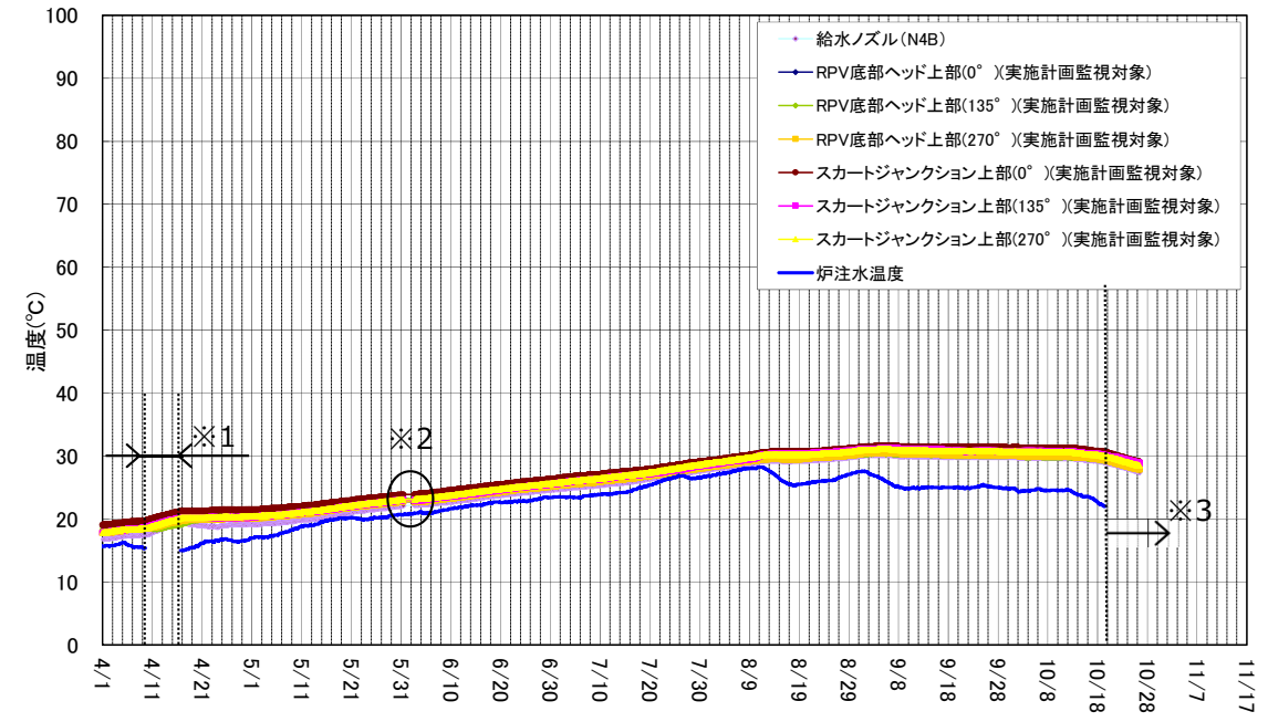
3号機 原子炉压力容器まわり温度 (4/1~10/26)
