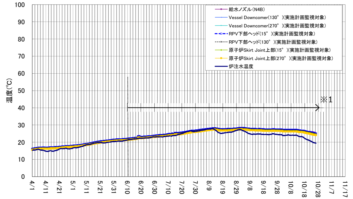
1号機 原子炉压力容器まわり温度(4/1~10/26)
