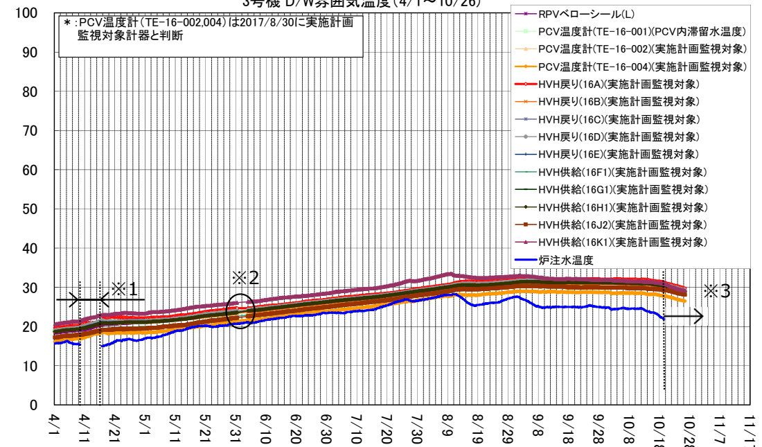
3号機 D/W雰囲気温度 (4/1~10/26)
