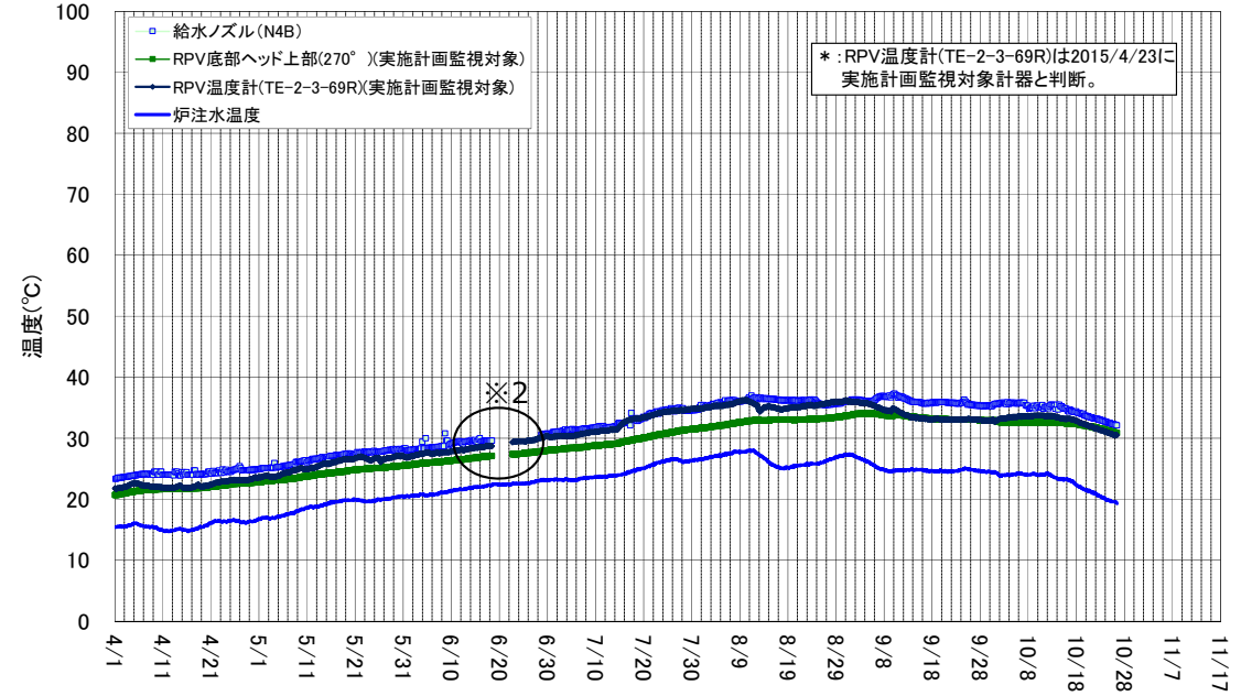
2号機 原子炉压力容器まわり温度 (4/1~10/26)
