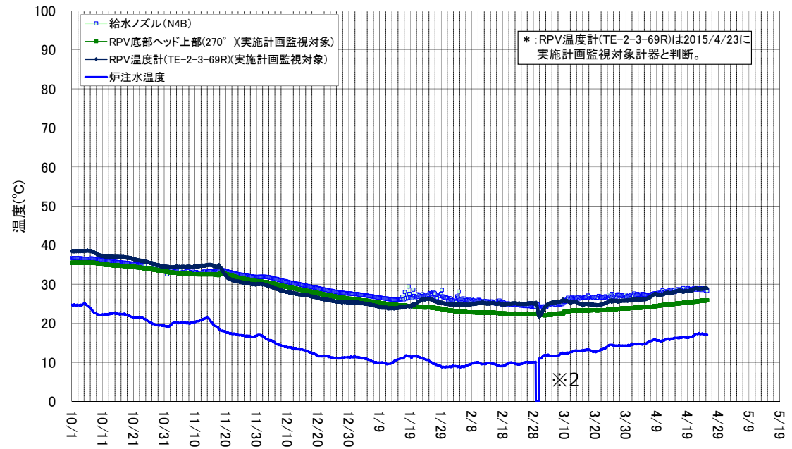
2号機 原子炉圧力容器まわり温度(10/1~4/25)
