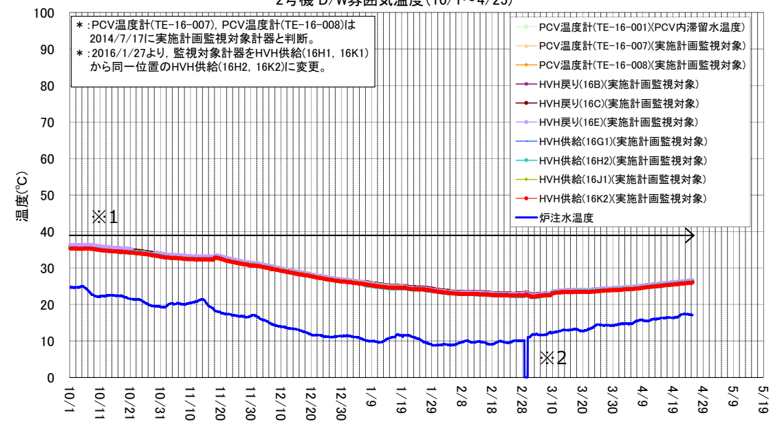
2号機 D/W雰囲気温度(10/1~4/25)
