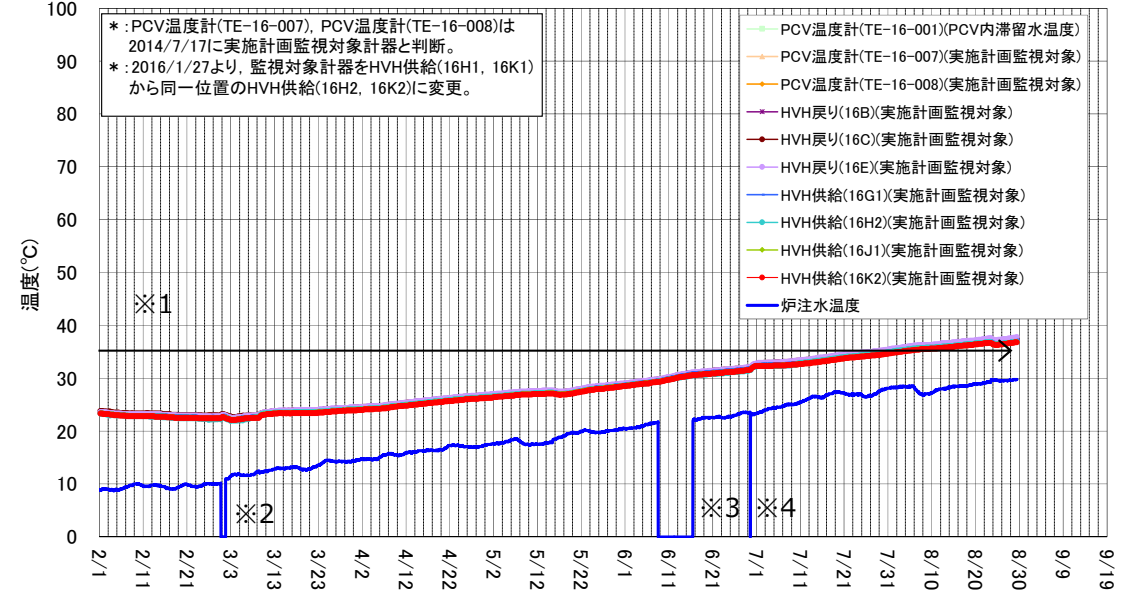
2号機 D/W雰囲気温度(2/1~8/29)
