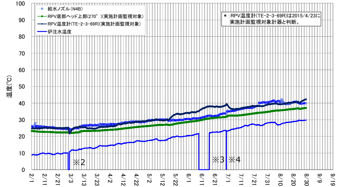
2号機 原子炉圧力容器まわり温度(2/1~8/29)
