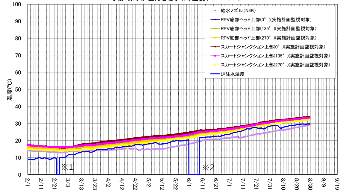
3号機 原子炉压力容器まわり温度(2/1~8/29)
