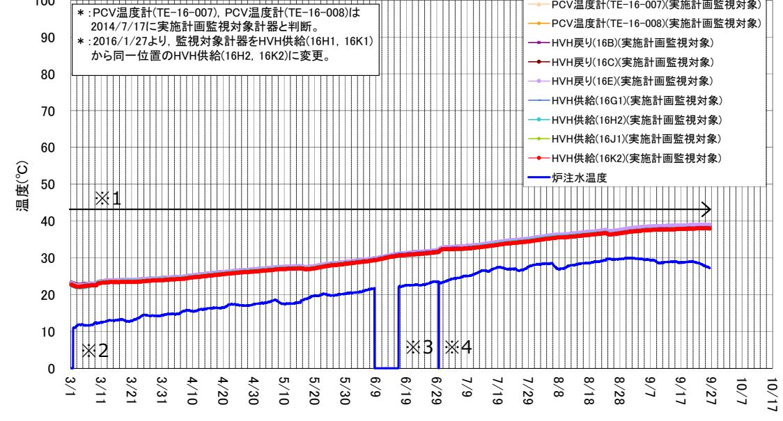
2号機 D/W雰囲気温度 (3/1~9/26)
