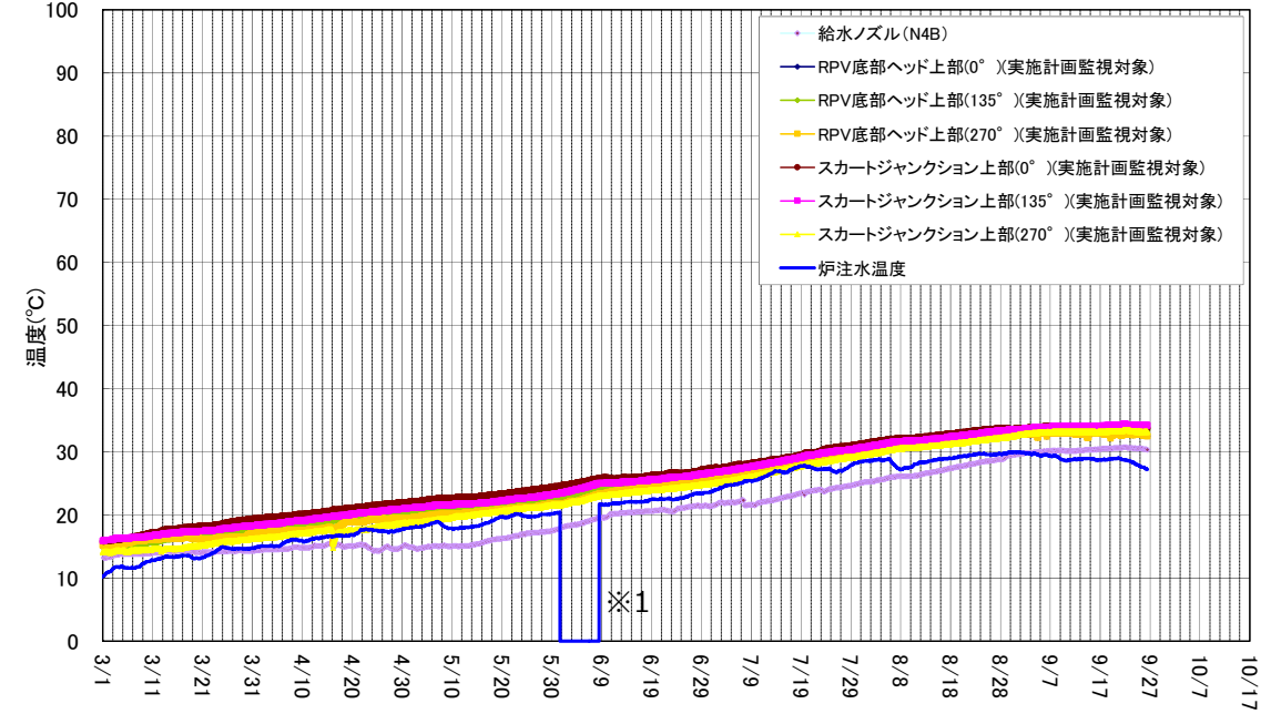
3号機 原子炉压力容器まわり温度 (3/1~9/26)
