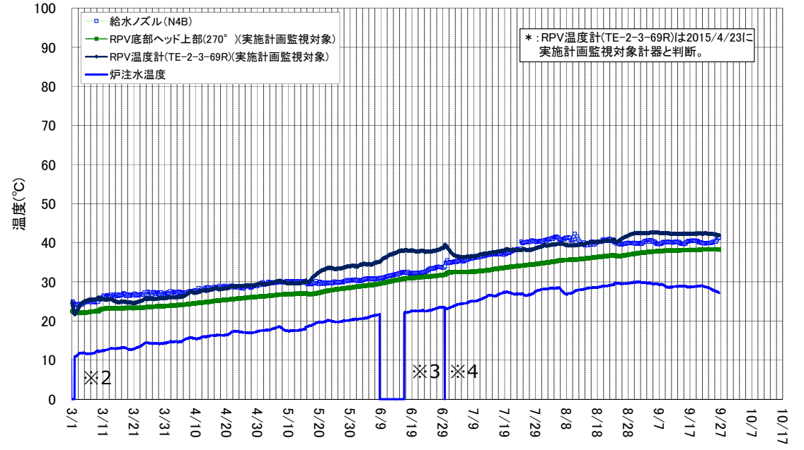
2号機 原子炉圧力容器まわり温度 (3/1~9/26)
