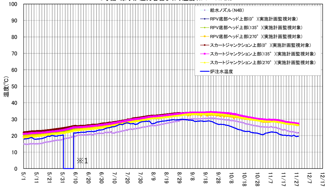
3号機 D/W雰囲気温度 (5/1~11/28)
