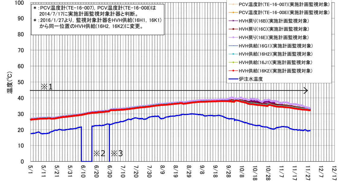
2号機 D/W雰囲気温度(5/1~11/28)
