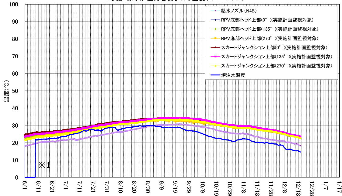
3号機 原子炉压力容器まわり温度(6/1~12/19)
