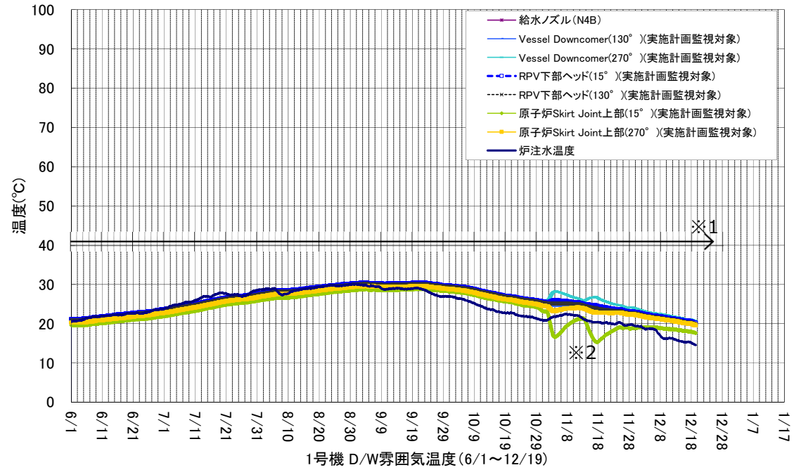
1号機 原子炉圧力容器まわり温度(6/1~12/19)
