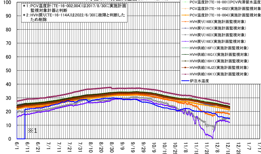
3号機 D/W雰囲気温度(6/1~12/19)
