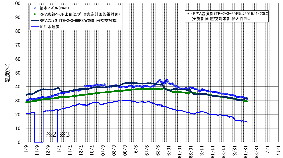
2号機 原子炉圧力容器まわり温度(6/1~12/19)
