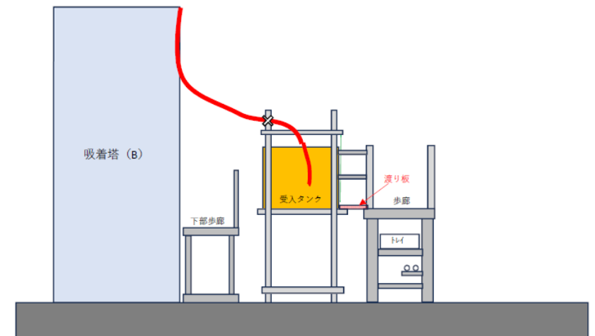
断面図 (A矢視)
