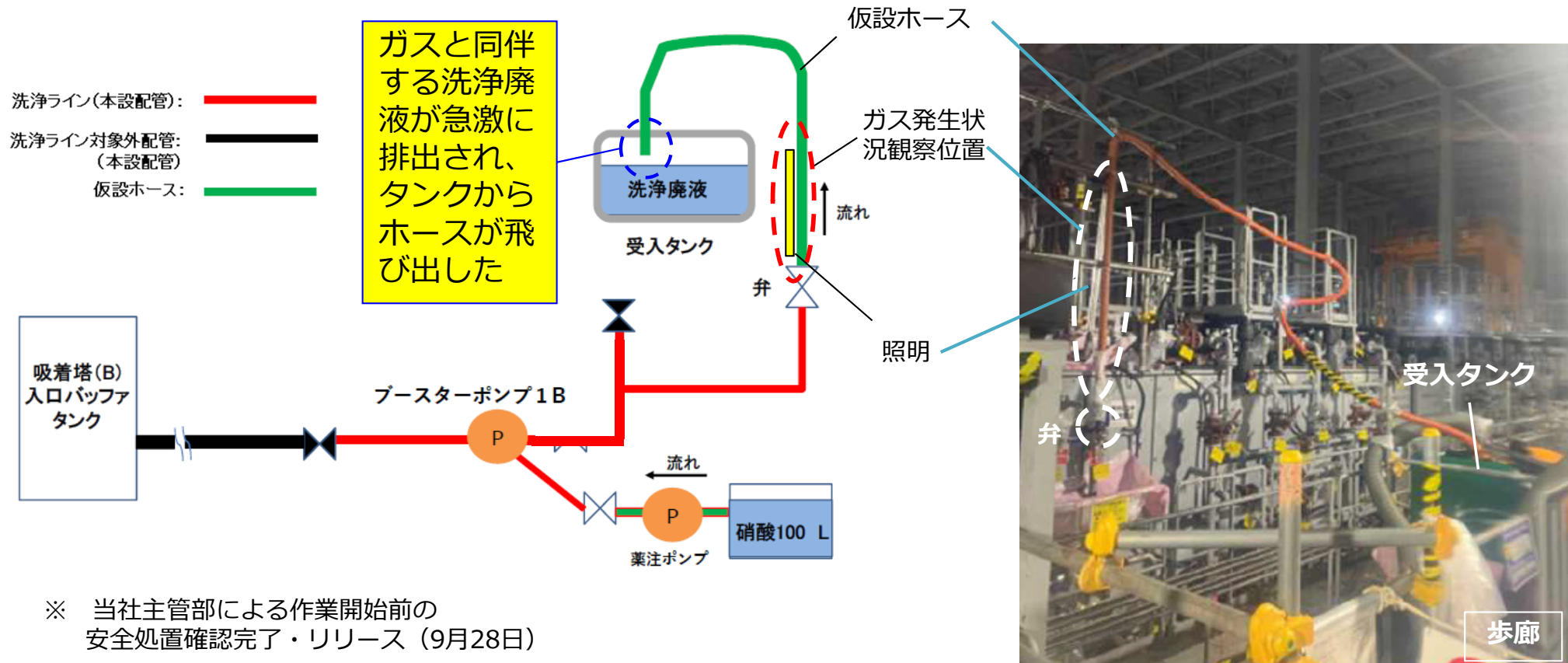
歩廊から吸着塔B側を見た写真
