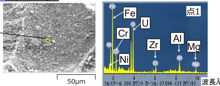
図3 微細混合相のSEM像及びWDX点分析スペクトル
