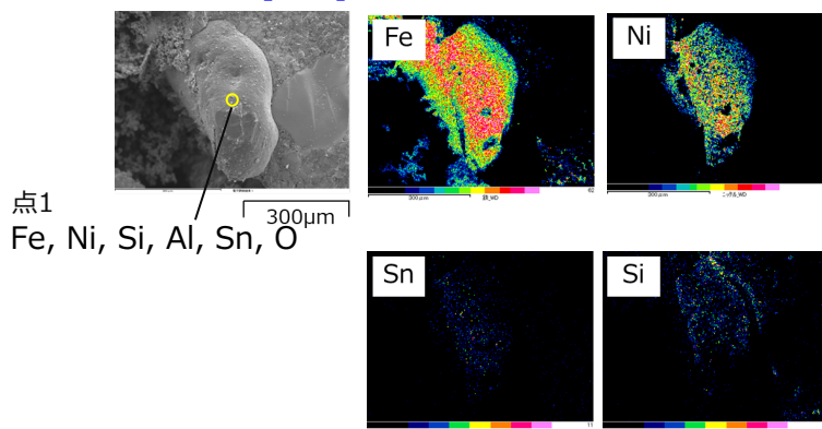
図3 SEM像及び元素マッピング
