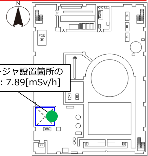
3号機R/B 3階
