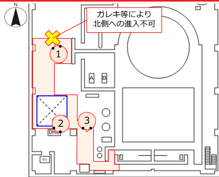
3号機R/B 3階
