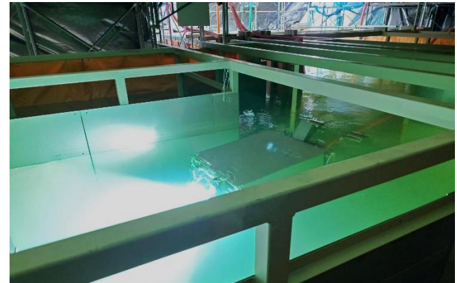
↑ 容器封入作業用ROVの遊泳試験の状況
