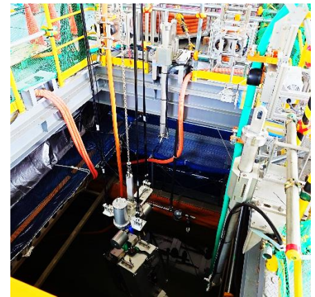
↑ 容器封入作業用ROVの投入
