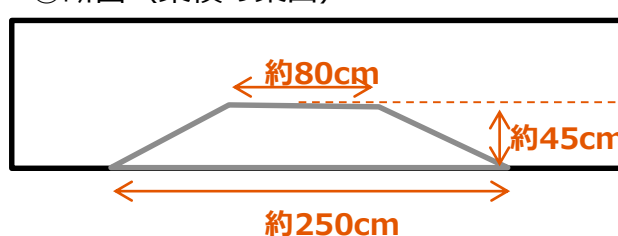
④断面（集積の築山）
