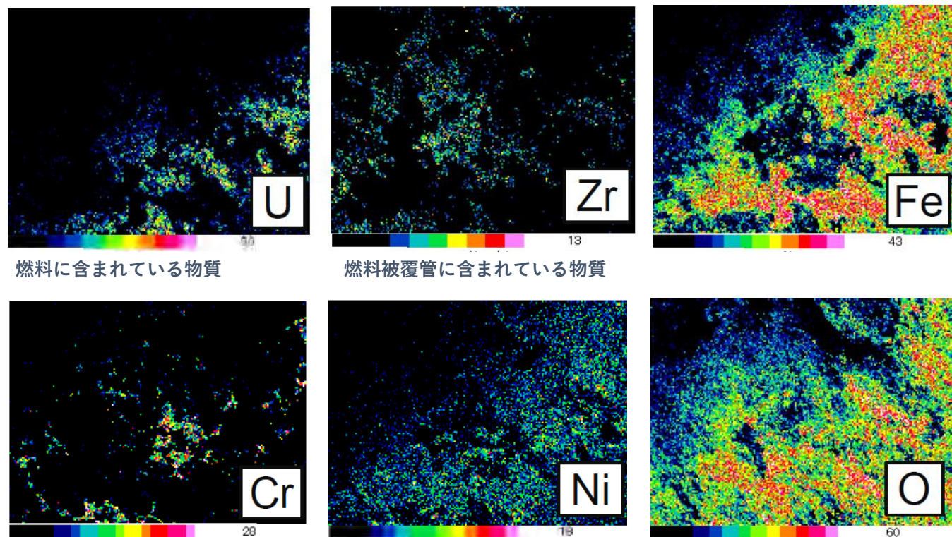
燃料デブリの波長分散型X線分析※2 (WDX) の 面分析測定結果
