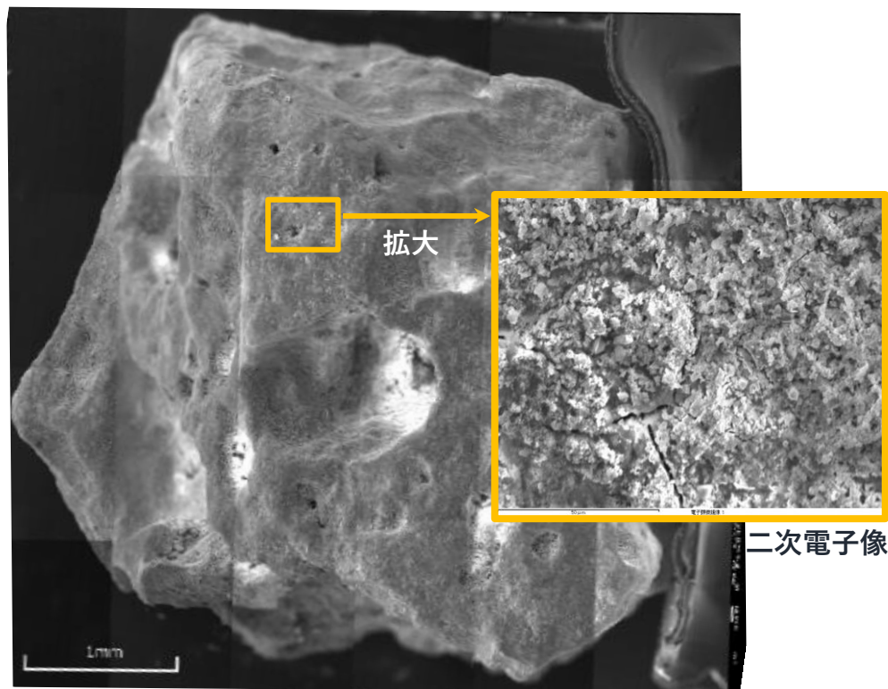
燃料デブリの走査型電子顕微鏡※1 (SEM) 観察結果
