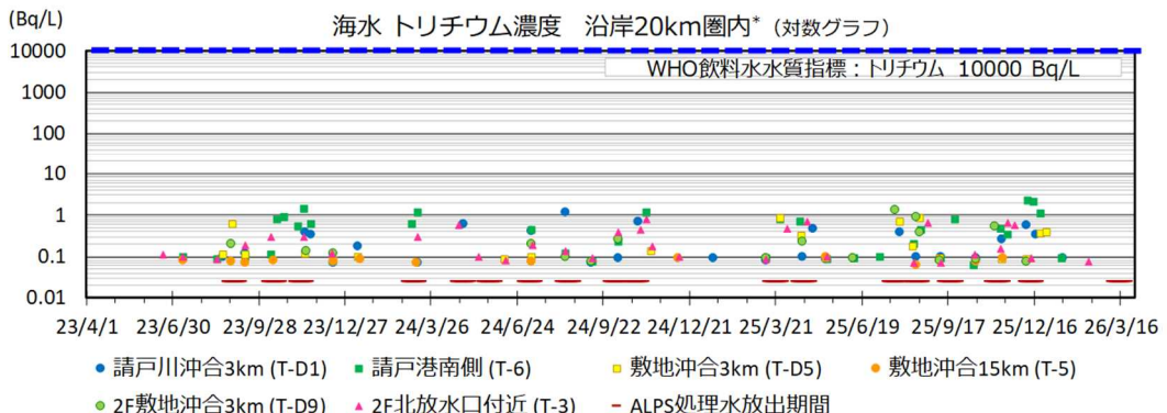
図Ⅲ-1-4 港湾外 20km 圏内の海水中トリチウム濃度
