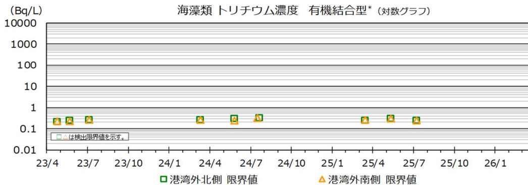
図Ⅲ-1-9 通常モニタリングの状況：海藻類 ～有機結合同型トリチウム～
