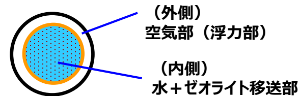
二重ホース断面図
