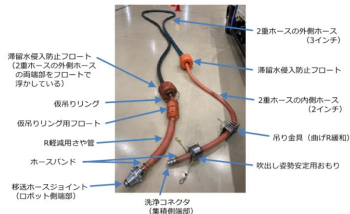
【参考】移送ホース（試験用）の全景写真
