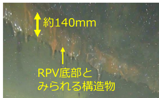
RPV底部とみられる構造物の厚さ
