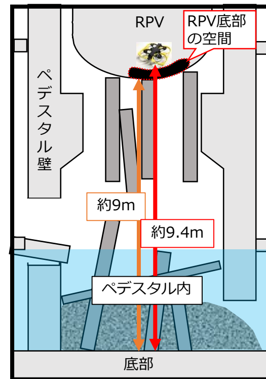
ドローンの飛行高さイメージ ペデスタル内 縦断面図
