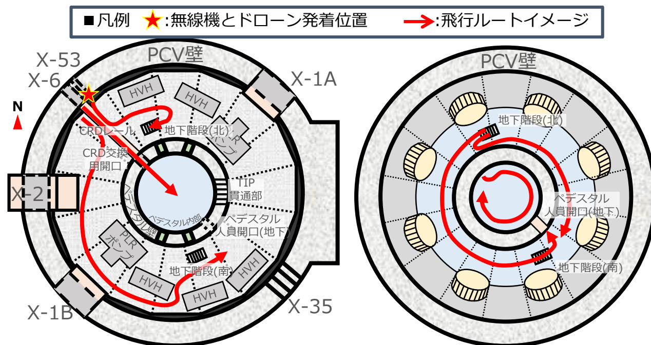
3号機 D/W 1FL 平面概略図
