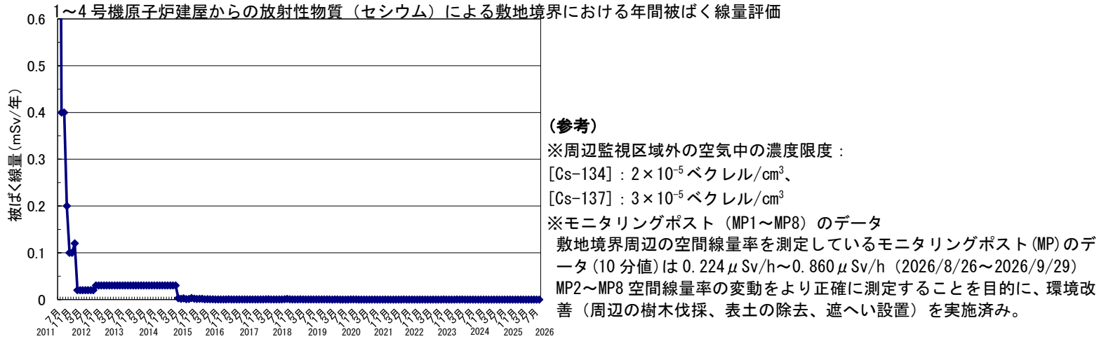
1～4 号機原子炉建屋からの放射性物質（セシウム）による敷地境界における年間被ばく線量評価
