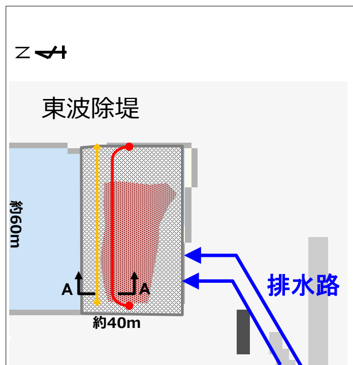
集積エリア平面図
