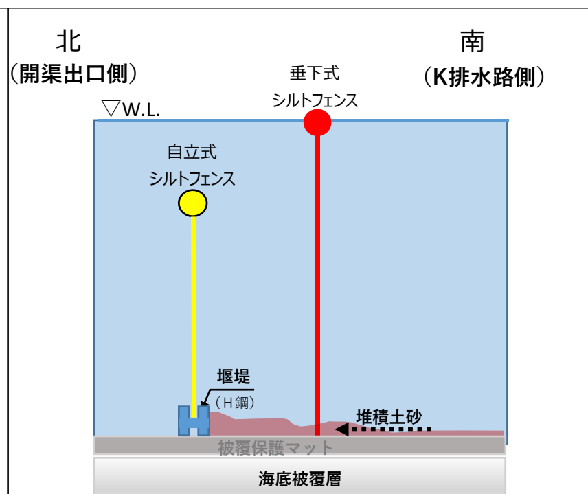
集積エリア断面図 (A-A)
