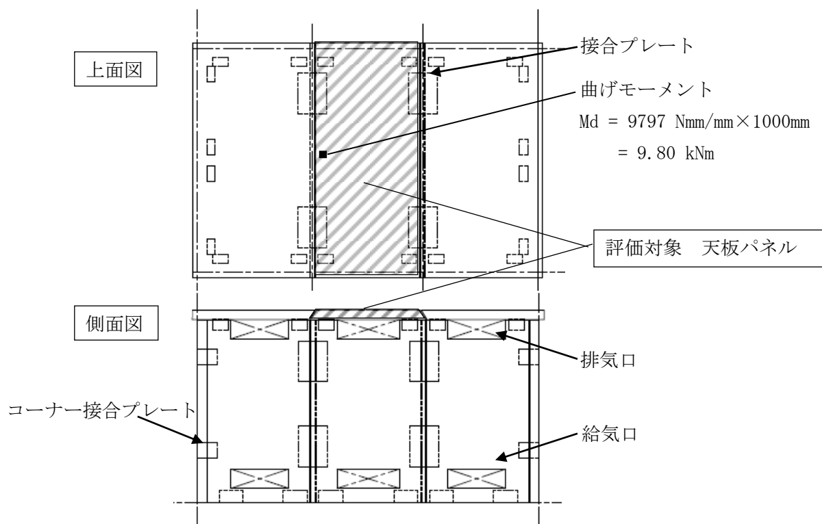
図 2.3-17 天板パネル
