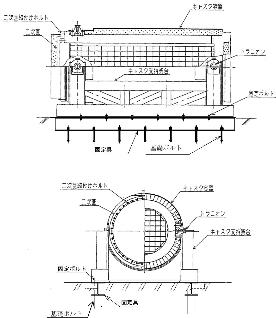
図 2.1-2 乾式貯蔵キャスクの概略構造図
