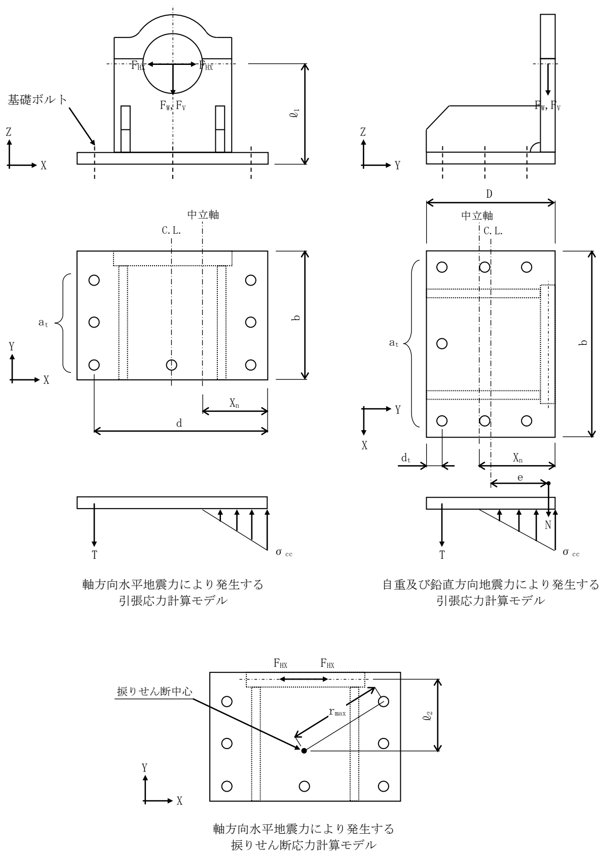
図 2.2-18 計算モデル図 (基礎ボルト)
