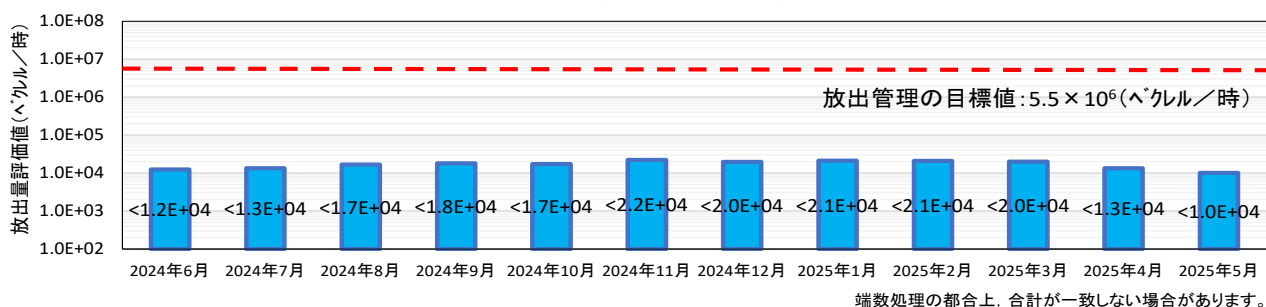
1号機 原子炉建屋、PCVガス管理システムからの放出量推移
