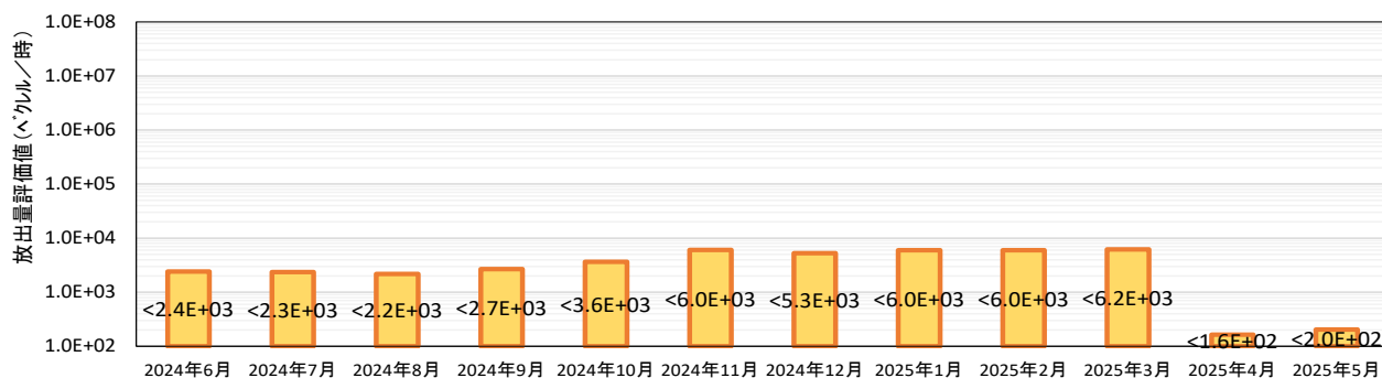
3号機 原子炉建屋、PCVガス管理システムからの放出量推移
