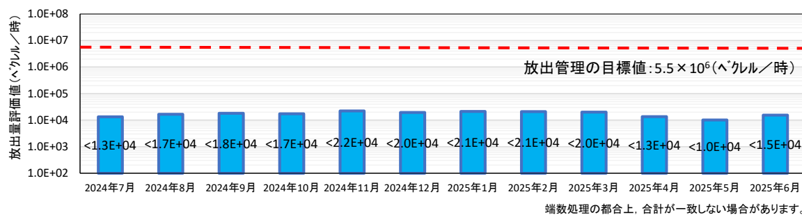
1号機 原子炉建屋、PCVガス管理システムからの放出量推移
