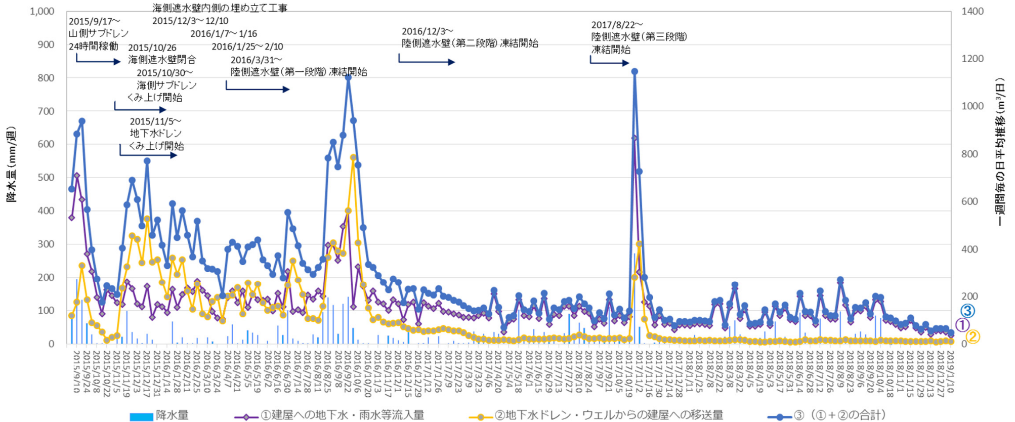
地下水ドレンからタービン建屋への移送量 ( 2019年1月3日 ~ 2019年1月9日 )
