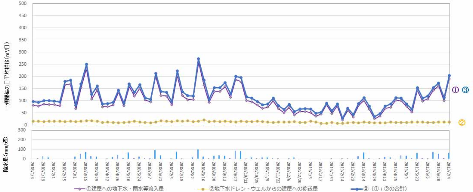
地下水ドレンからタービン建屋への移送量 ( 2019年6月27日 ~ 2019年7月3日 )
