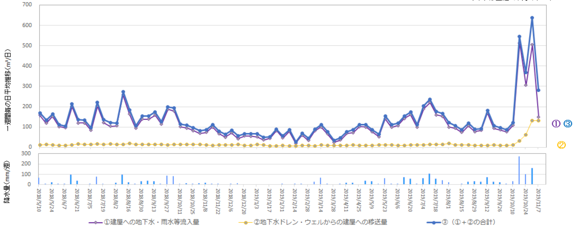
地下水ドレンからタービン建屋への移送量 (2019年10月31日 ~ 2019年11月6日)
