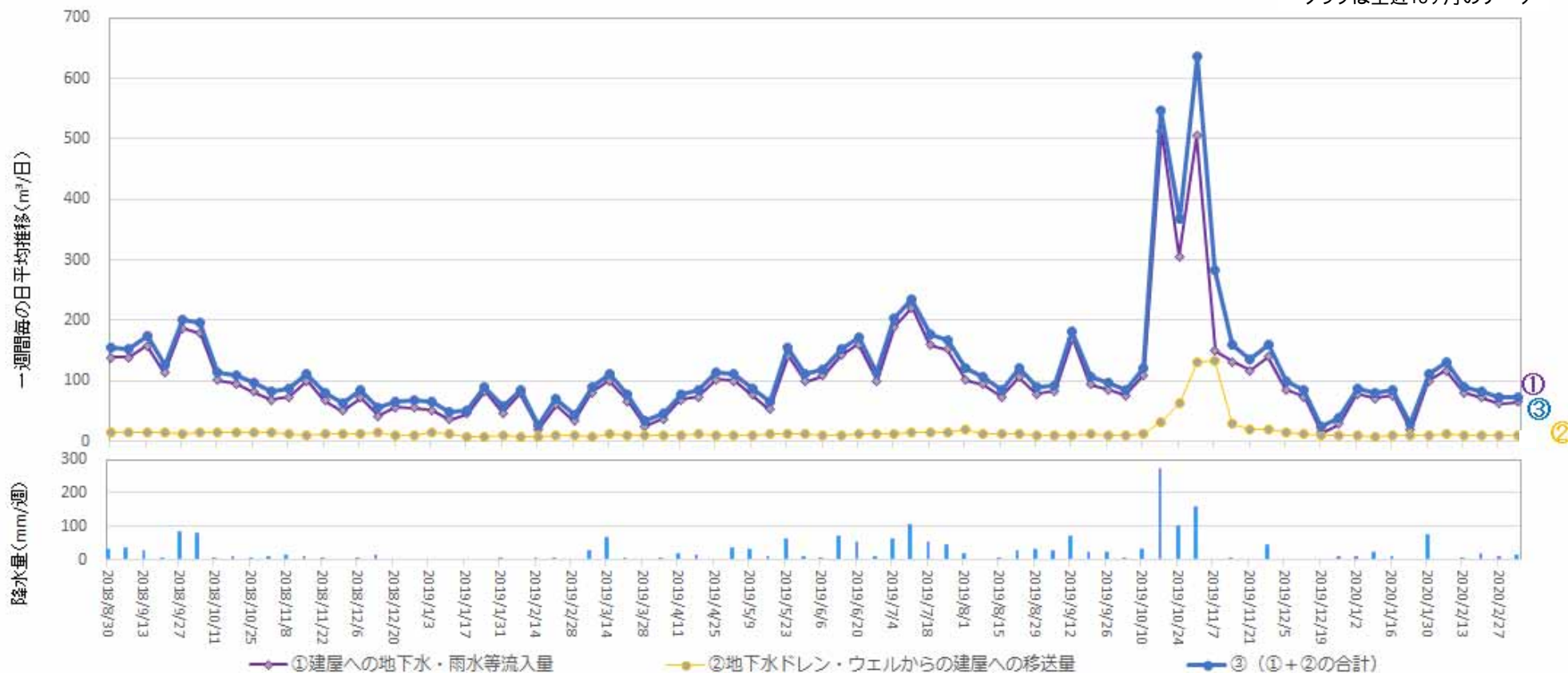
地下水ドレンからタービン建屋への移送量 ( 2020年2月27日 ~ 2020年3月4日 )
