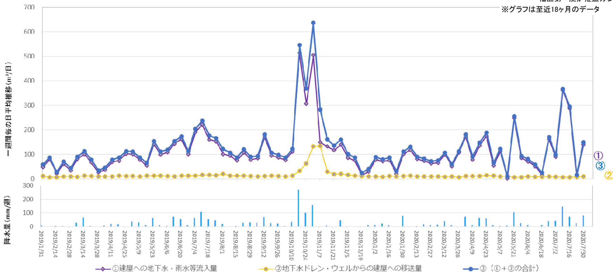
地下水ドレンからタービン建屋への移送量 (2020年7月23日 ~ 2020年7月29日)
