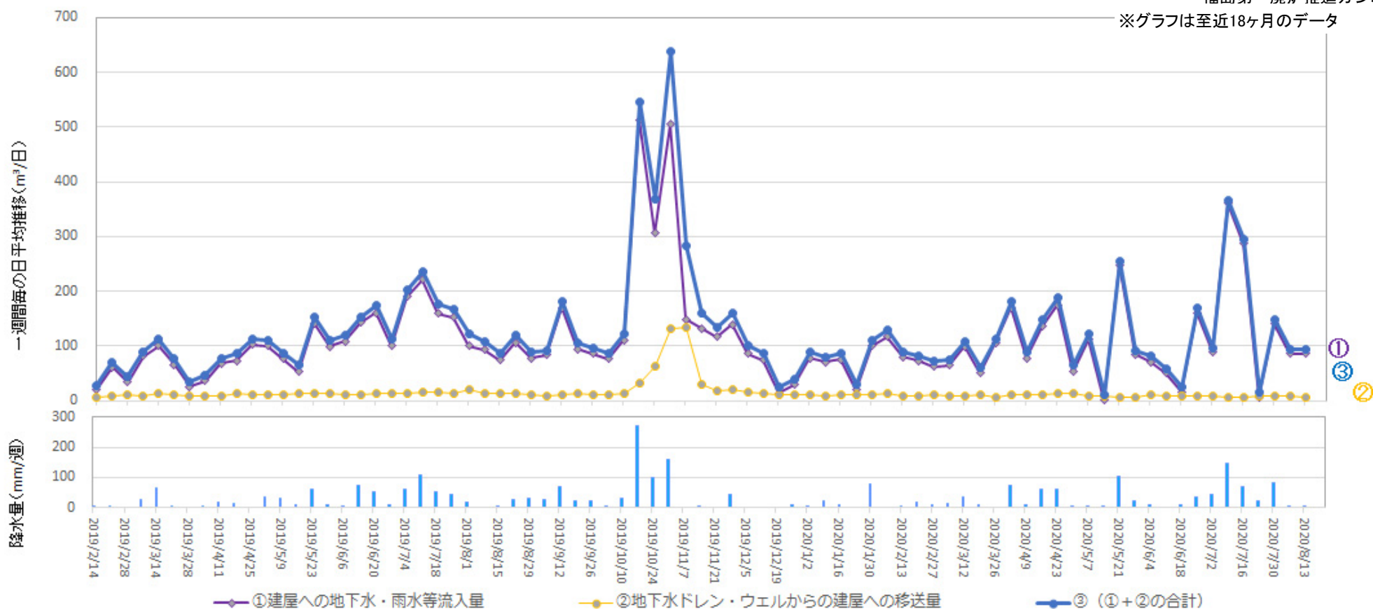
地下水ドレンからタービン建屋への移送量 (2020年8月6日 ~ 2020年8月12日)
