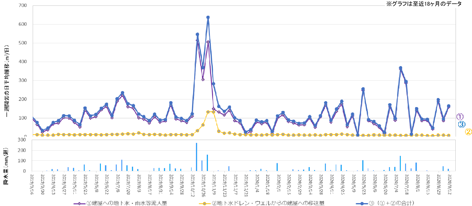
地下水ドレンからタービン建屋への移送量 (2020年9月3日 ~ 2020年9月9日)
