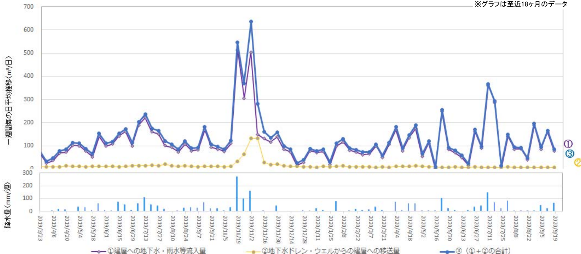
地下水ドレンからタービン建屋への移送量 (2020年9月10日 ~ 2020年9月16日)
