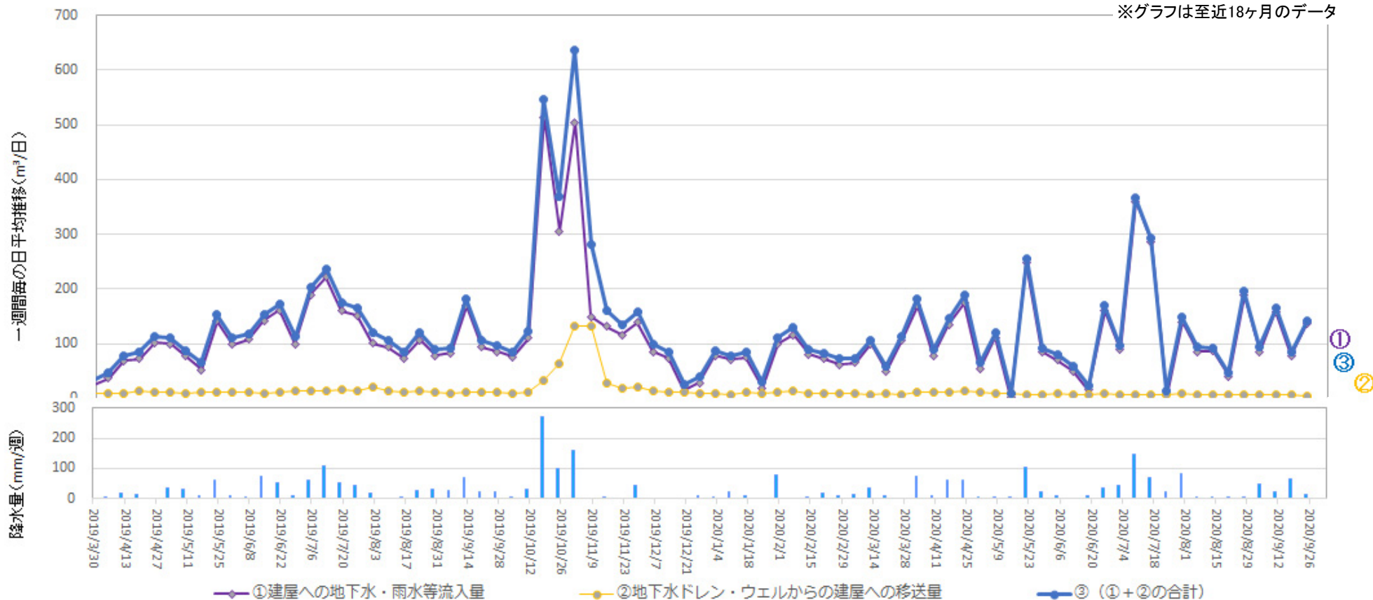
地下水ドレンからタービン建屋への移送量 (2020年9月17日 ~ 2020年9月23日)
