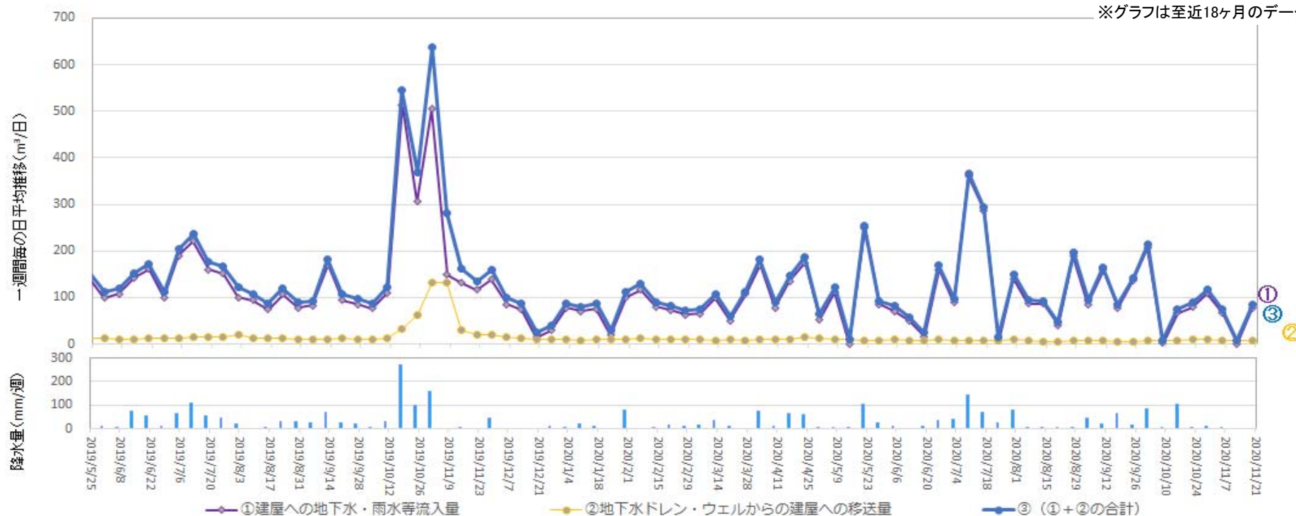
地下水ドレンからタービン建屋への移送量 (2020年11月12日 ~ 2020年11月18日)
