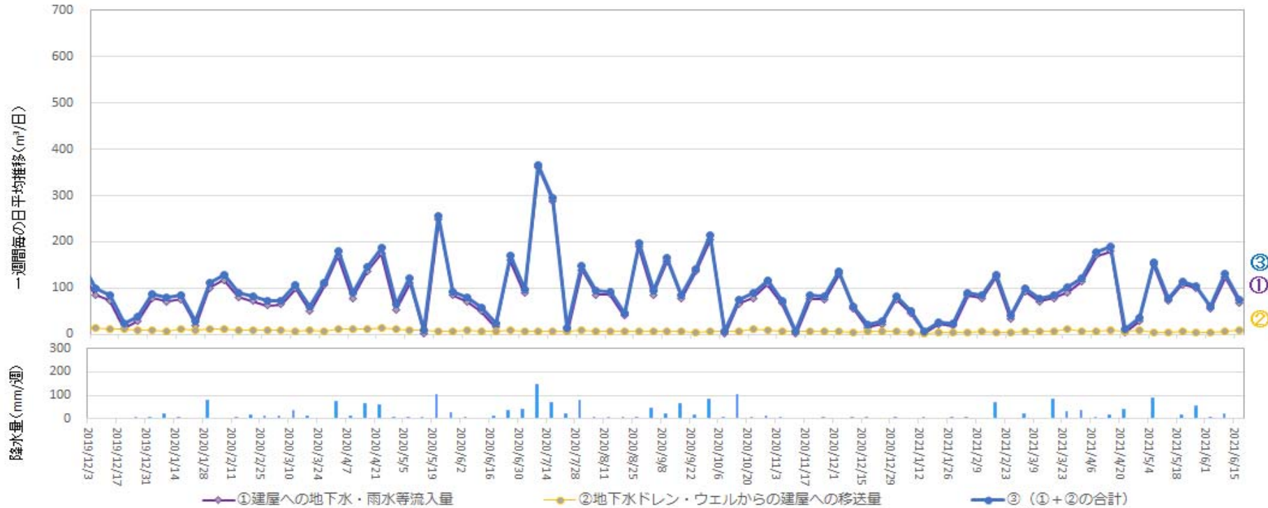
地下水ドレンからタービン建屋への移送量 ( 2021年6月10日 ~ 2021年6月16日 )
