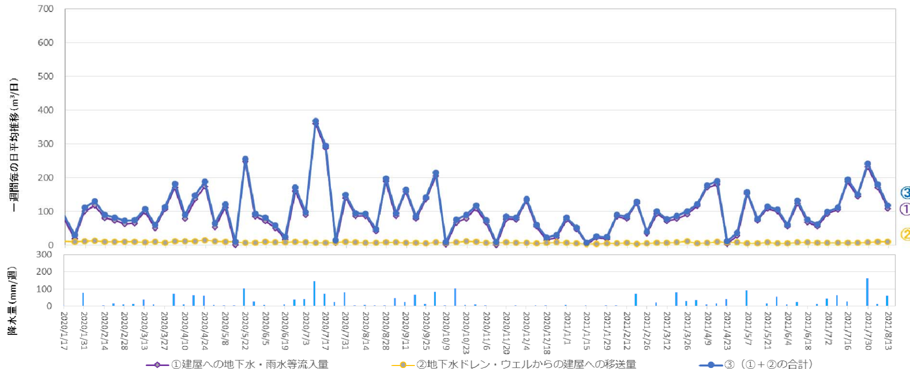
地下水ドレンからタービン建屋への移送量 ( 2021年8月5日 ~ 2021年8月11日 )
