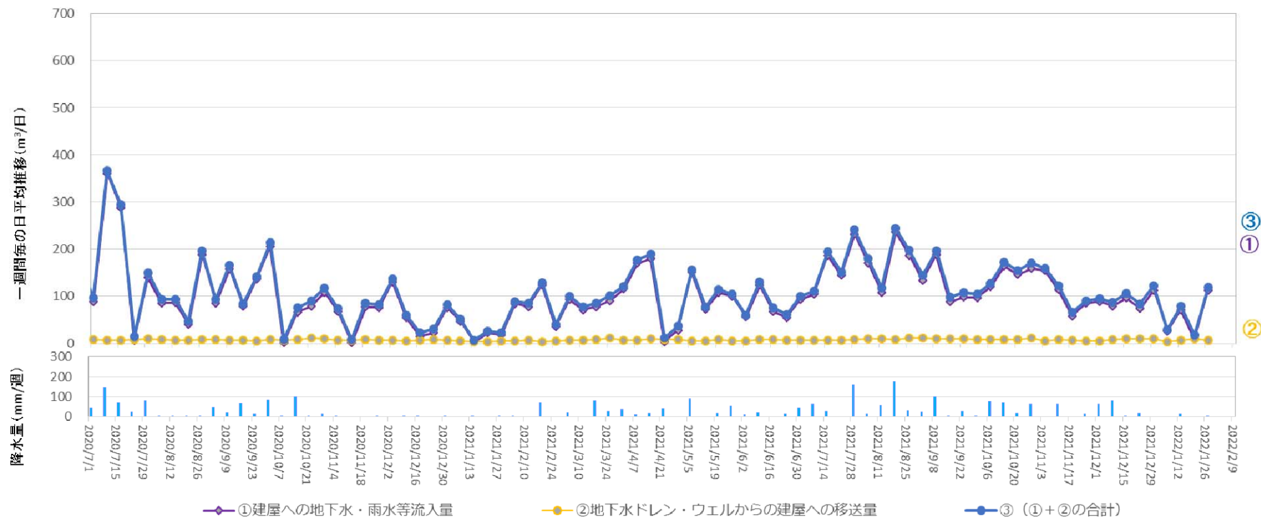
地下水ドレンからタービン建屋への移送量 ( 2022年1月20日 ~ 2022年1月26日 )
