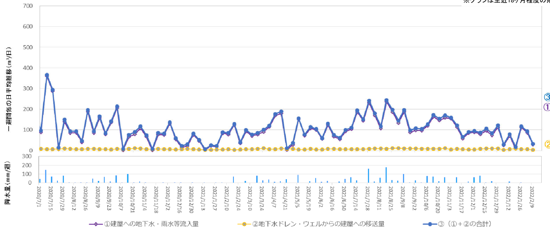
地下水ドレンからタービン建屋への移送量 ( 2022年2月3日 ~ 2022年2月9日 )
