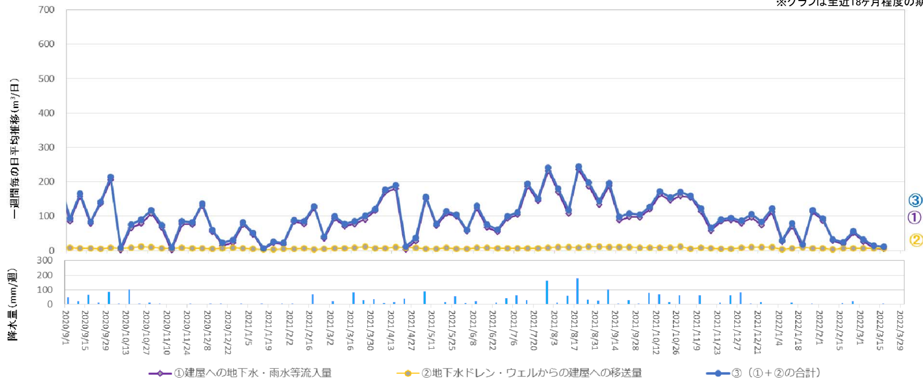
地下水ドレンからタービン建屋への移送量 ( 2022年3月10日 ~ 2022年3月16日 )
