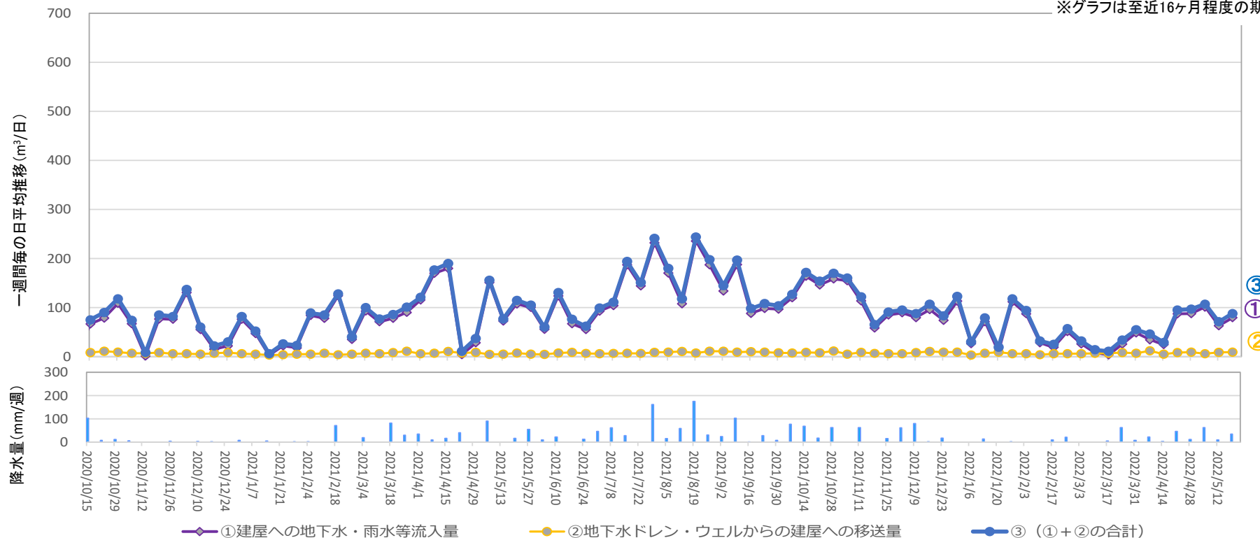
地下水ドレンからタービン建屋への移送量 ( 2022年5月12日 ~ 2022年5月18日 )
