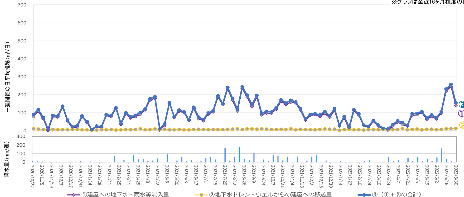
地下水ドレンからタービン建屋への移送量 ( 2022年6月16日 ~ 2022年6月22日 )
