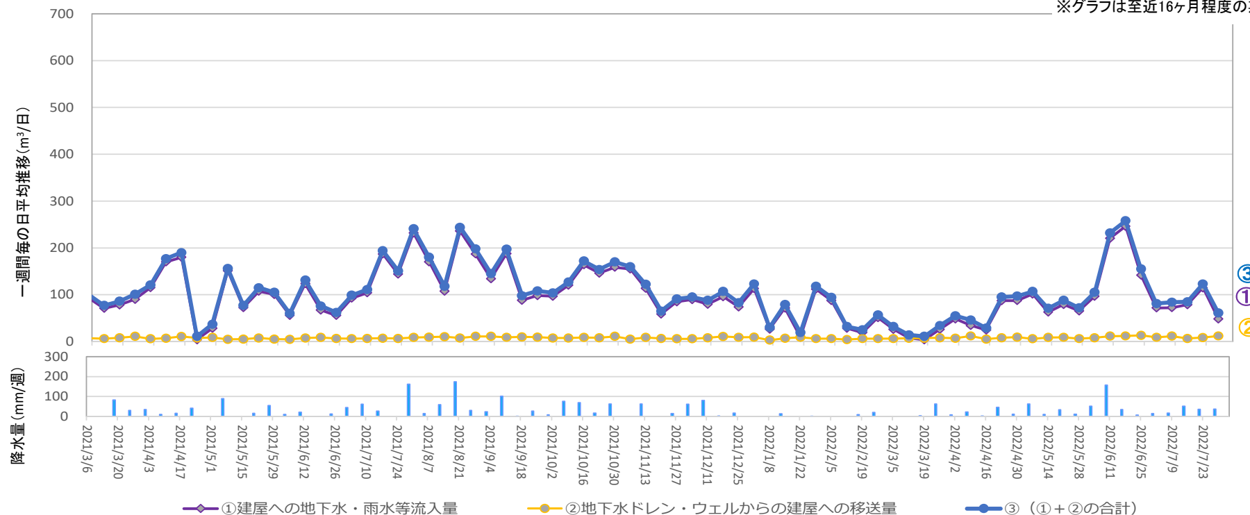
地下水ドレンからタービン建屋への移送量 ( 2022年7月21日 ~ 2022年7月27日 )
