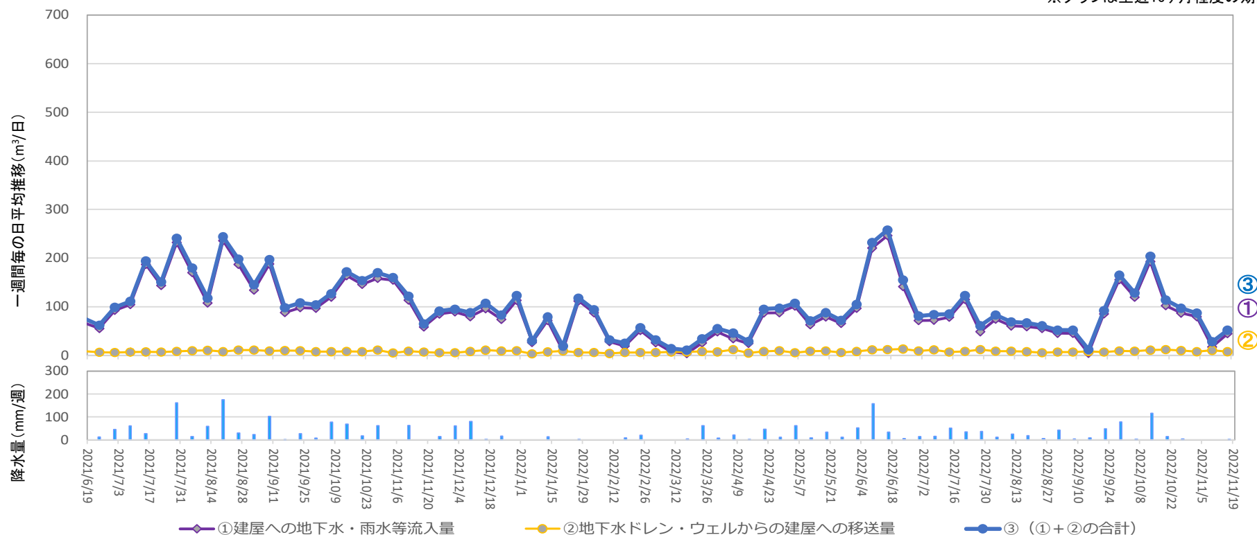
地下水ドレンからタービン建屋への移送量 (2022年11月10日 ~ 2022年11月16日)
