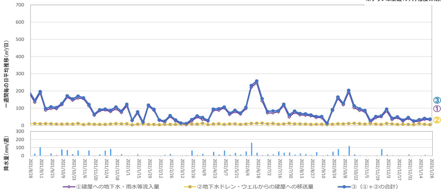
地下水ドレンからタービン建屋への移送量 ( 2023年1月19日 ~ 2023年1月25日 )
