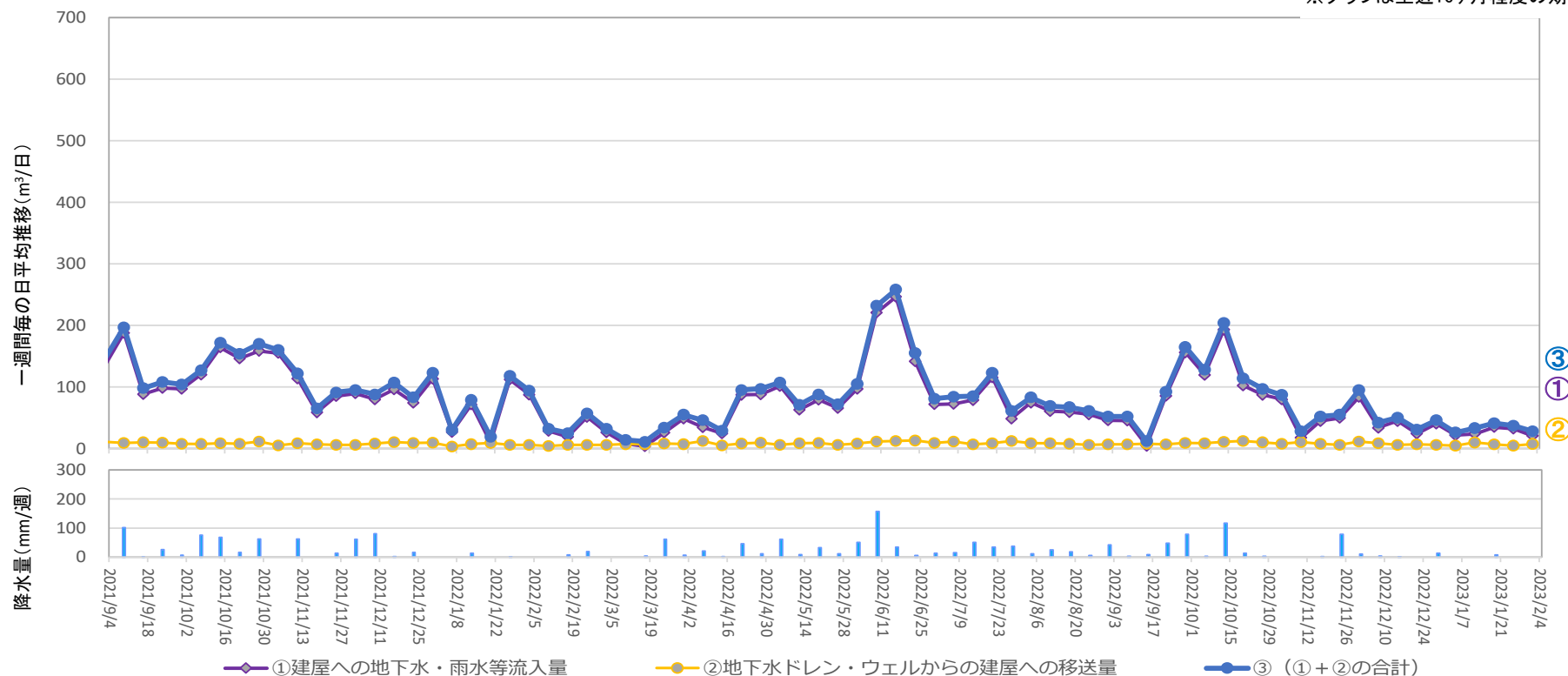
地下水ドレンからタービン建屋への移送量 ( 2023年1月26日 ~ 2023年2月1日 )
