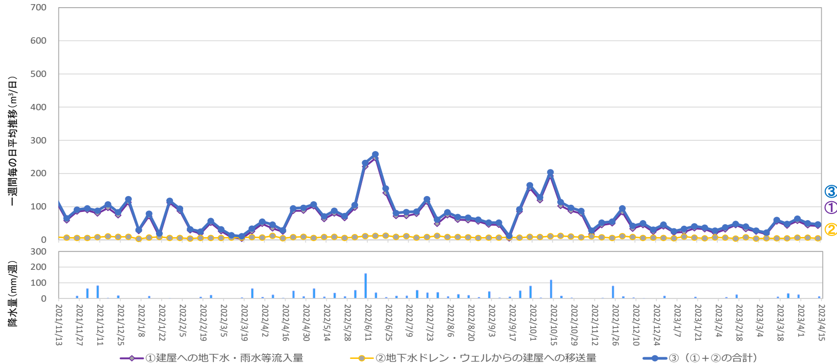
地下水ドレンからタービン建屋への移送量 ( 2023年4月6日 ~ 2023年4月12日 )
