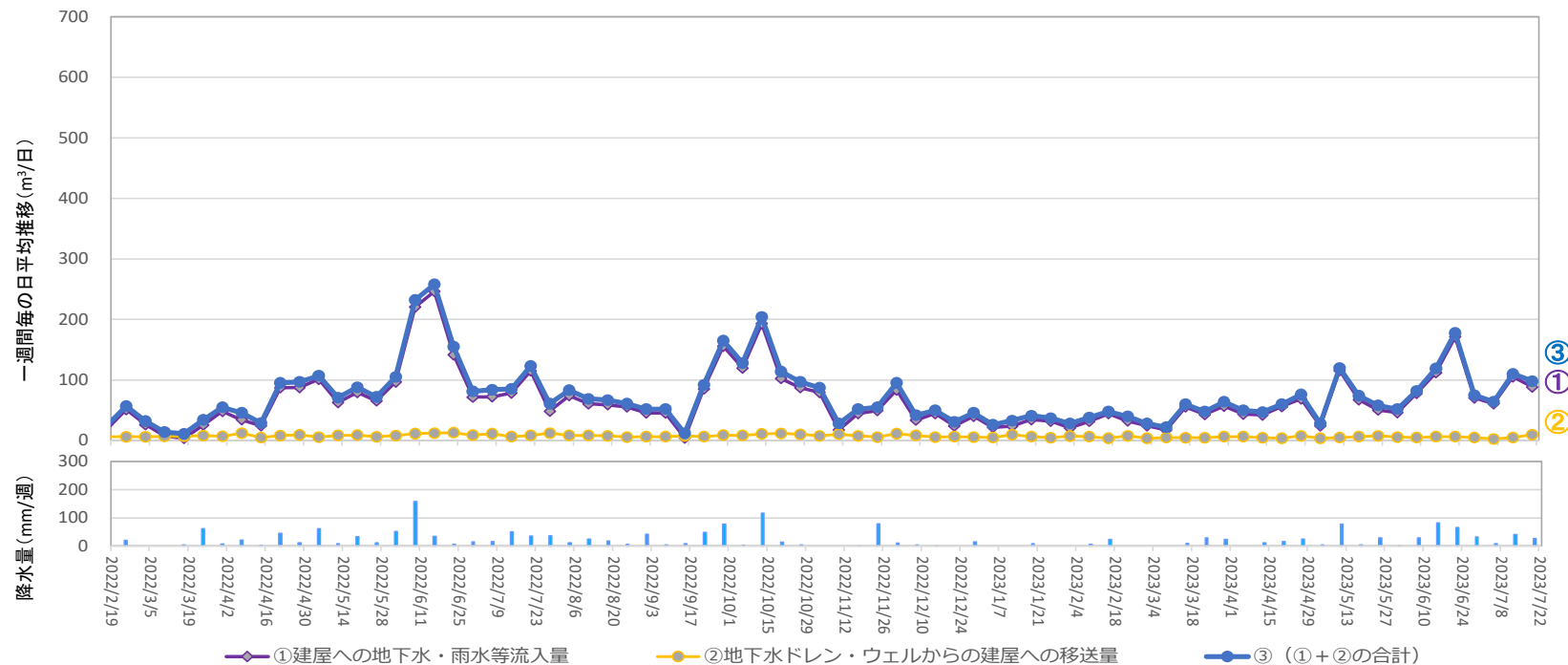
地下水ドレンからタービン建屋への移送量 ( 2023年7月13日 ~ 2023年7月19日 )
