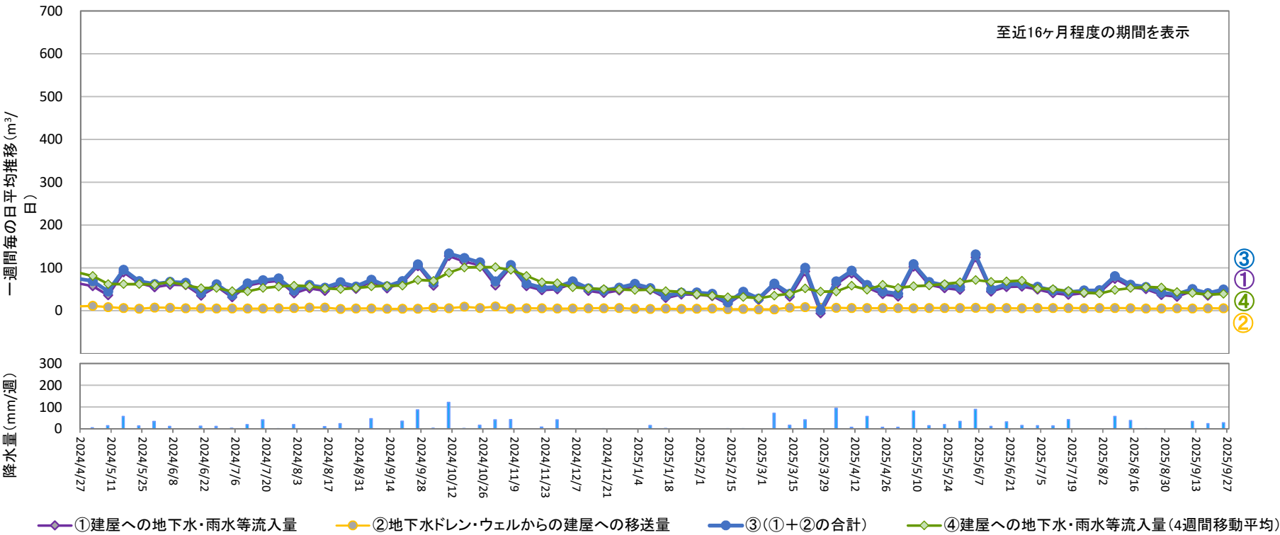
地下水ドレンからタービン建屋への移送量 ( 2025年9月18日 ～ 2025年9月24日 ) [m³／日]
