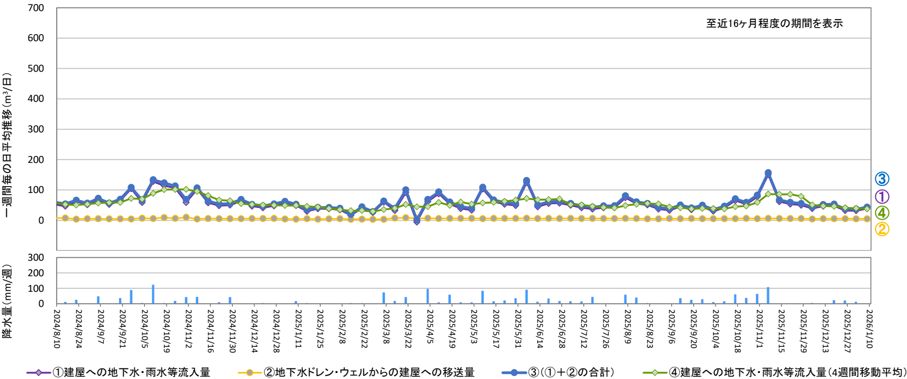
地下水ドレンからタービン建屋への移送量 ( 2026年1月1日 ~ 2026年1月7日 ) [m³／日]
