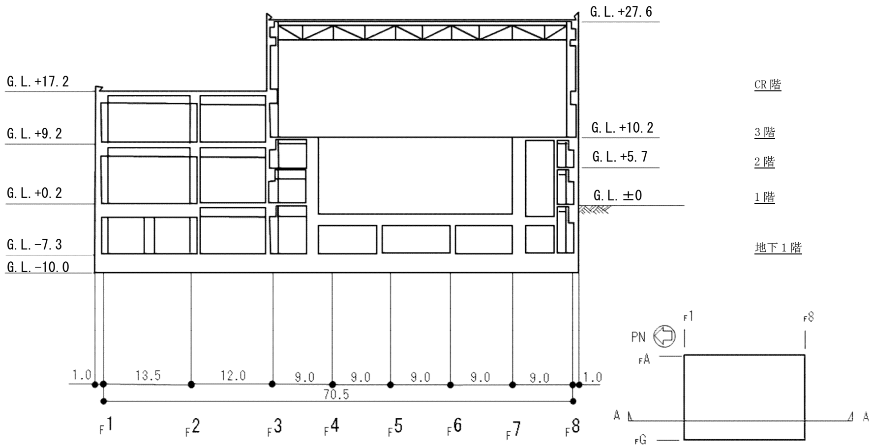
图1.2 PL/B NS方向断面图 (单位：m)
