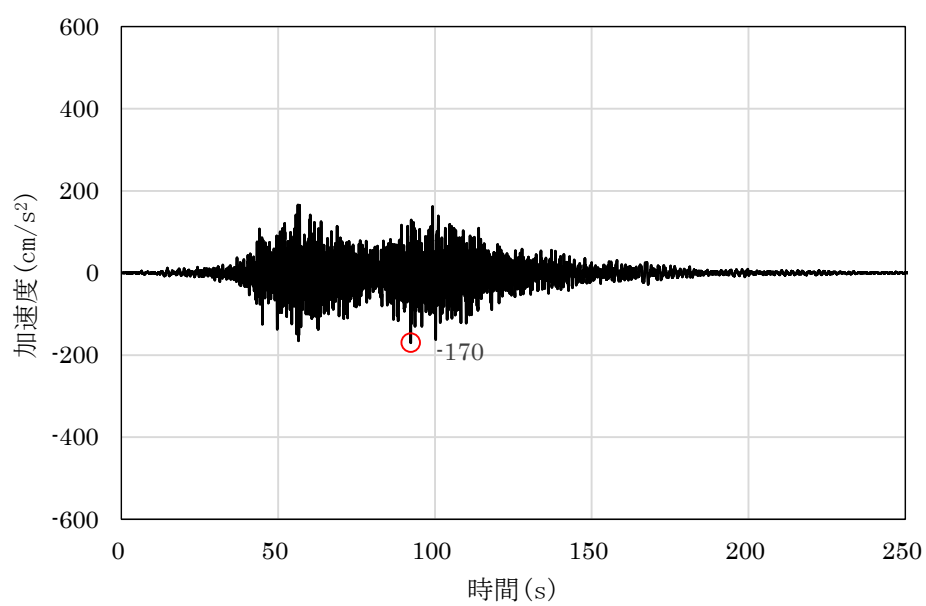
図－23 建屋の基礎底面位置における入力地震動の加速度時刻歴波形 (1/2Ss450-② 水平方向【EW 方向】)
