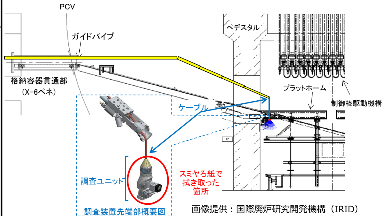
2号機PCV内部調査の概要（2018年1月実施）
