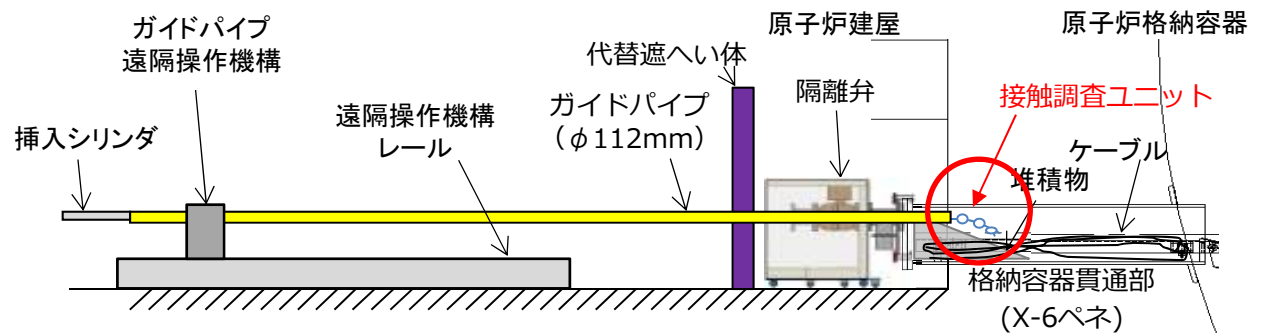
2号機原子炉格納容器貫通部内堆積物調査の概略
