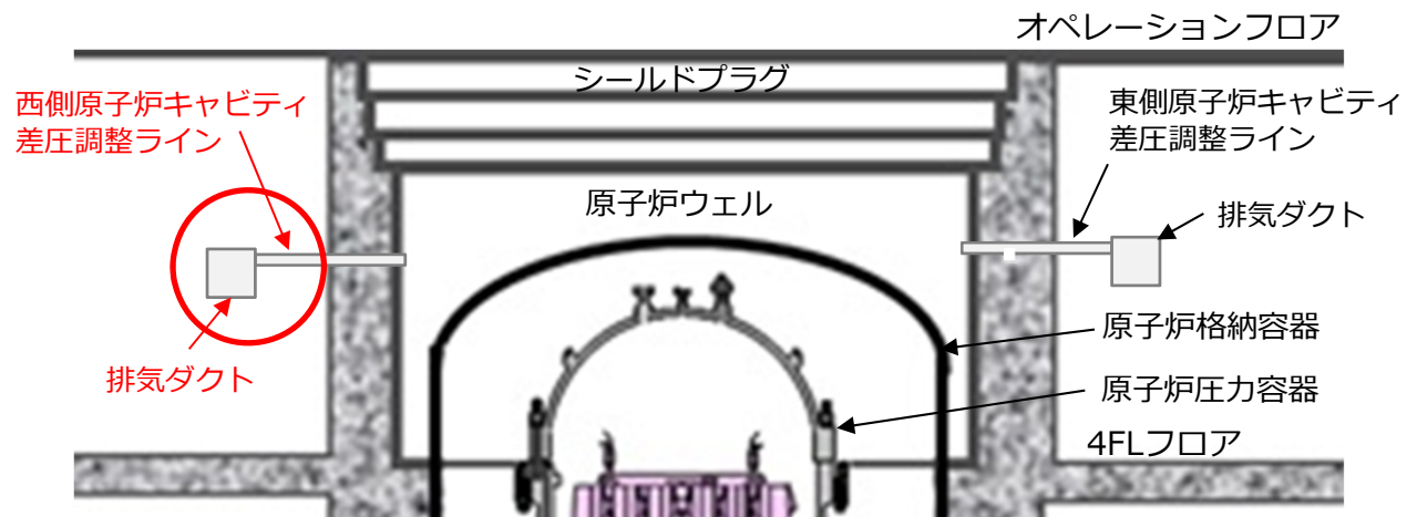
2号機原子炉キャビティ差圧調整ライン調査の概略
