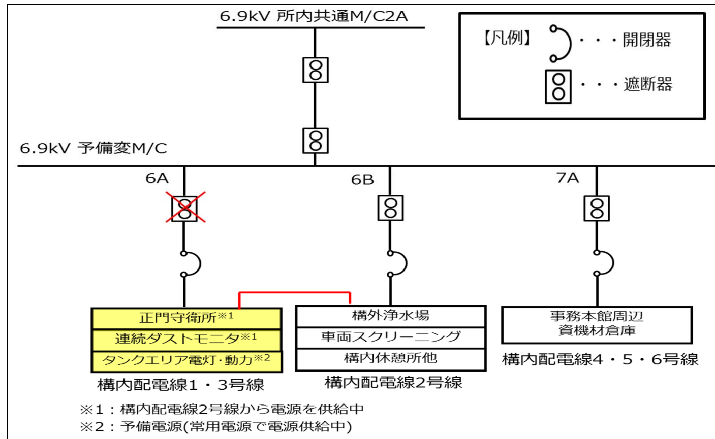
6.9KV予備変M/C(配電盤)過負荷トリップ警報発生に伴う影響範囲図
